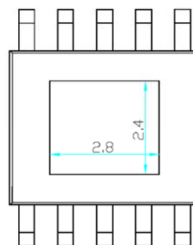
ESSOP10-8R底面图
