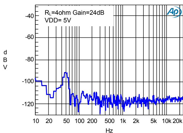
Noise FFT
